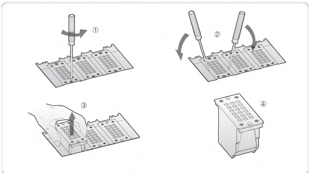
Рис. 7. Демонтаж дугогасительной камеры
