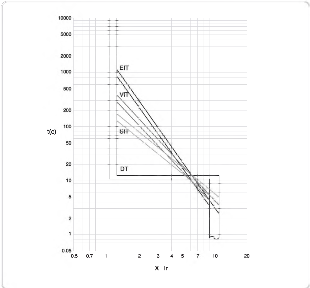
Рисунок 8. Характеристики IDMTL
