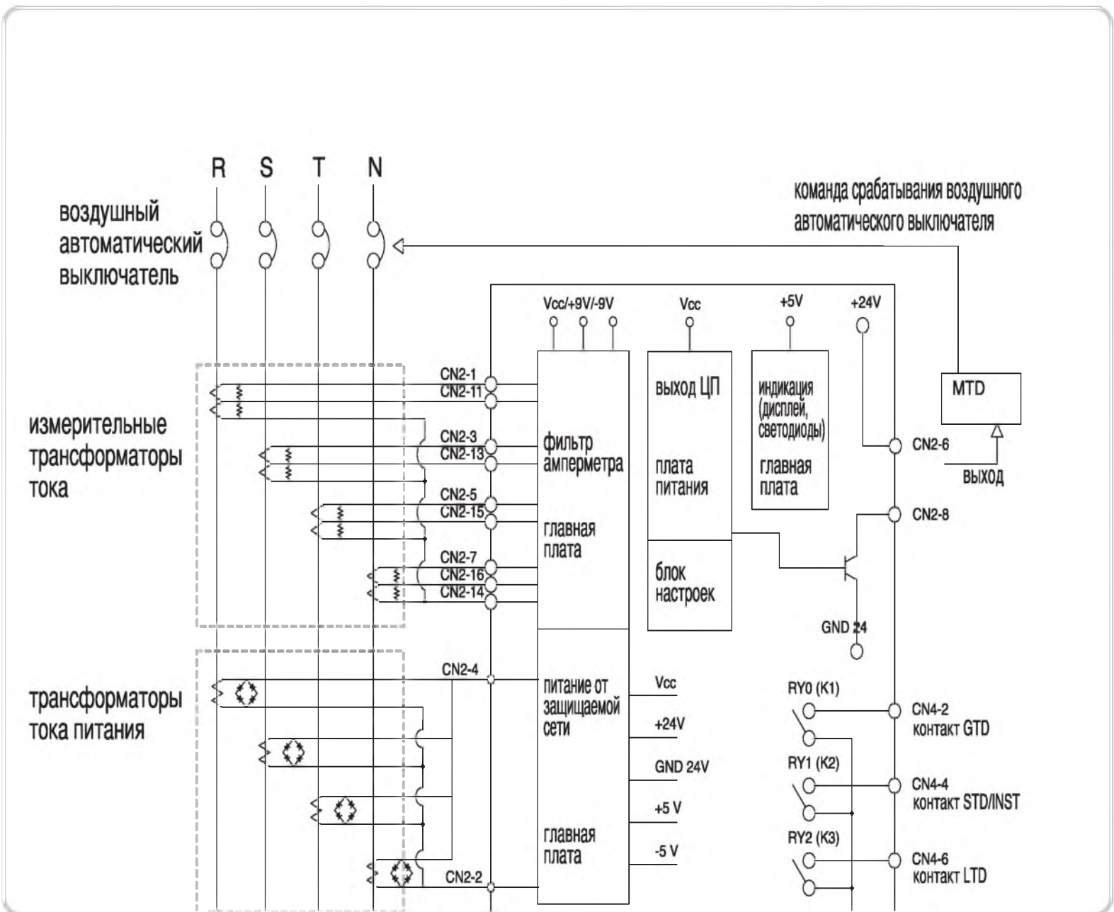
■ Схема подключений
