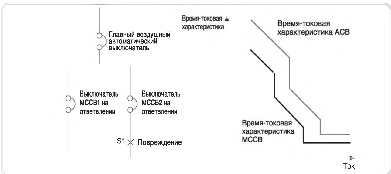
Рис. 2. Селективная защита
