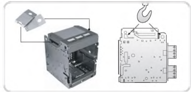
Рис. 3. Подъем выкатного выключателя
