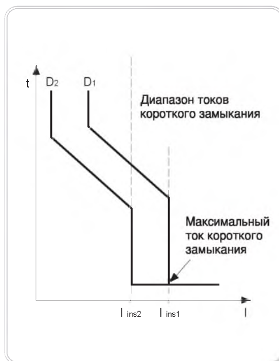
Рисунок 3. Токковая селективность
